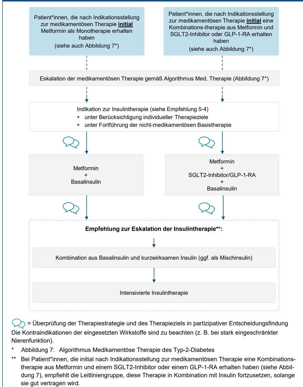
Abbildung 8: Algorithmus Insulintherapie
